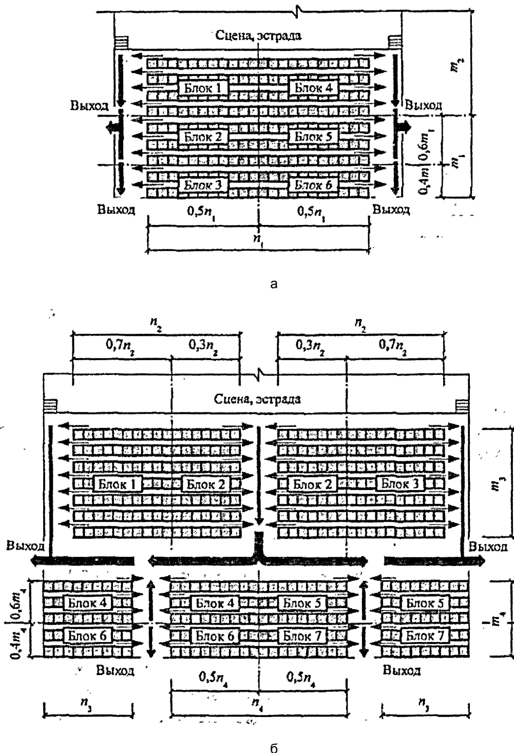
Рисунок Ж.1. Маршрутизация движения людских потоков при эвакуации из зрительных залов а - с боковыми (продольными) проходами; б - с поперечным проходом
